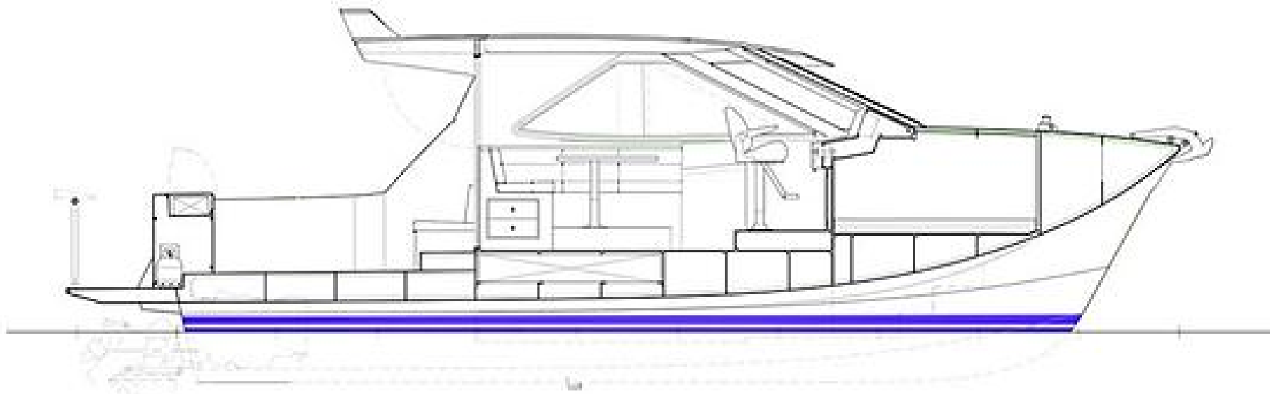
LONGITUDINAL SECTION
